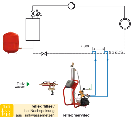
Beispiel: Einkesselanlage
