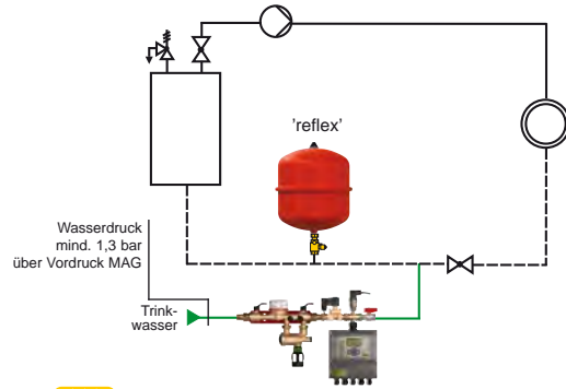
Beispiel: Heizungsanlage
